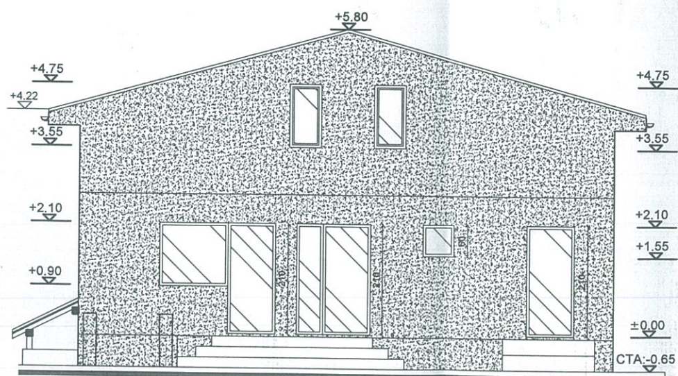
fatada posterioara
