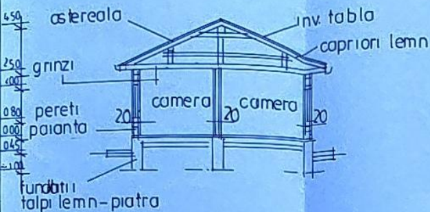
● SÈCTIUNE (A-A) 1:100
