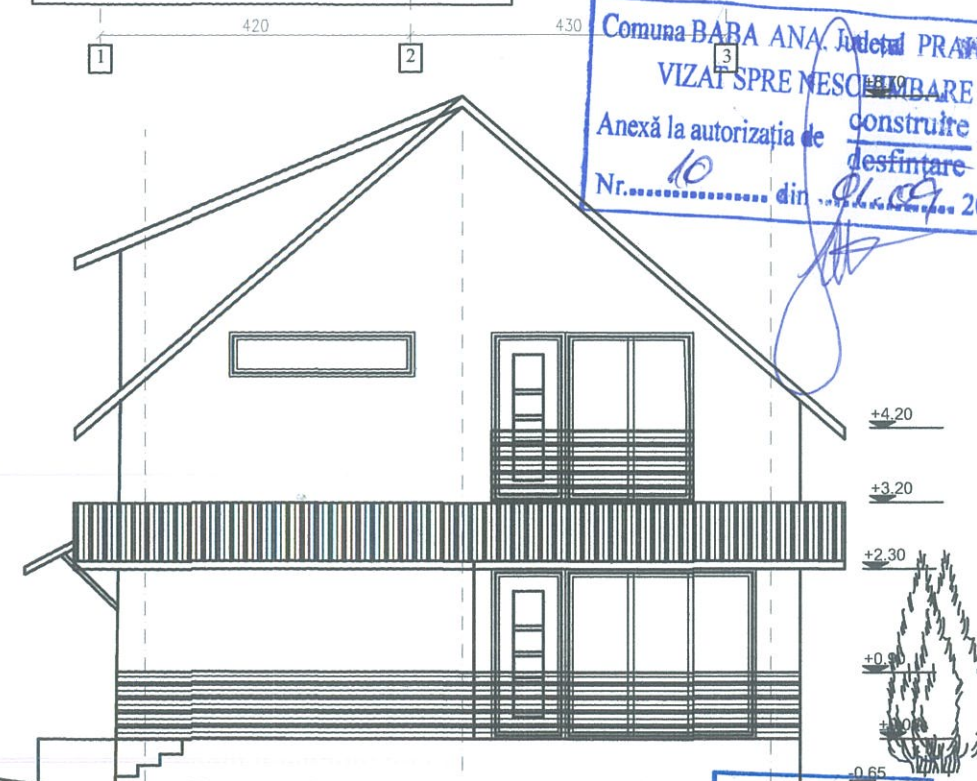
FATADA POSTERIOARA, Scara 1:100
