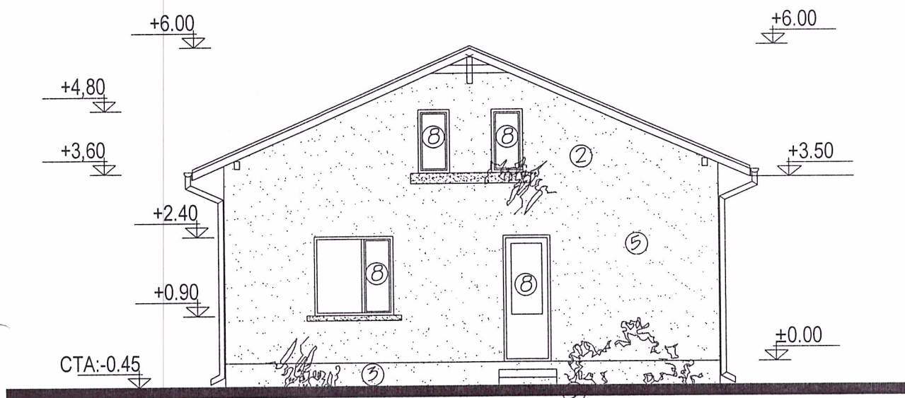
FATADA POSTERIOARA SC 1:100
